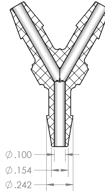
SECTION A-A
