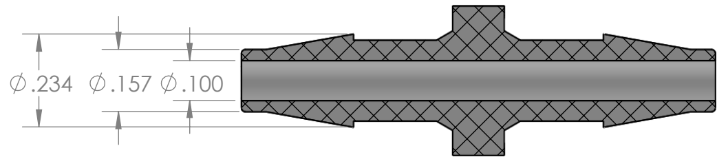
SECTION A-A
