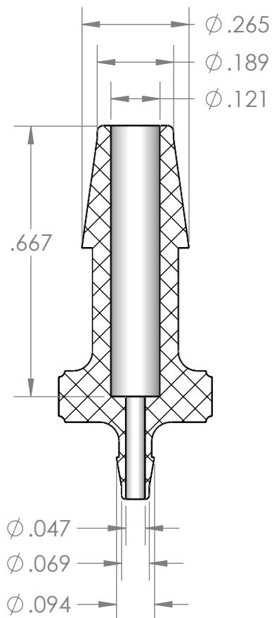
SECTION A-A
