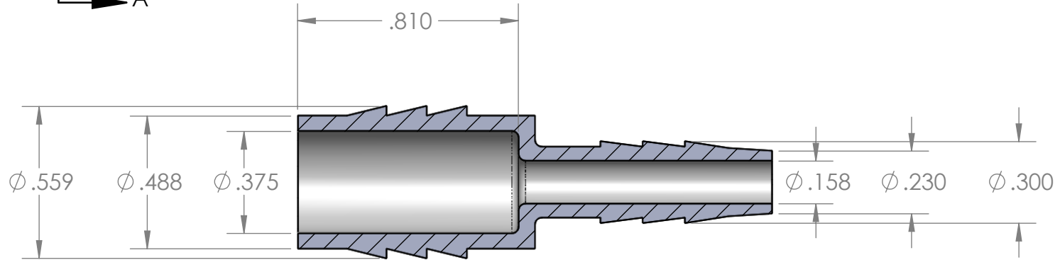
SECTION A-A
