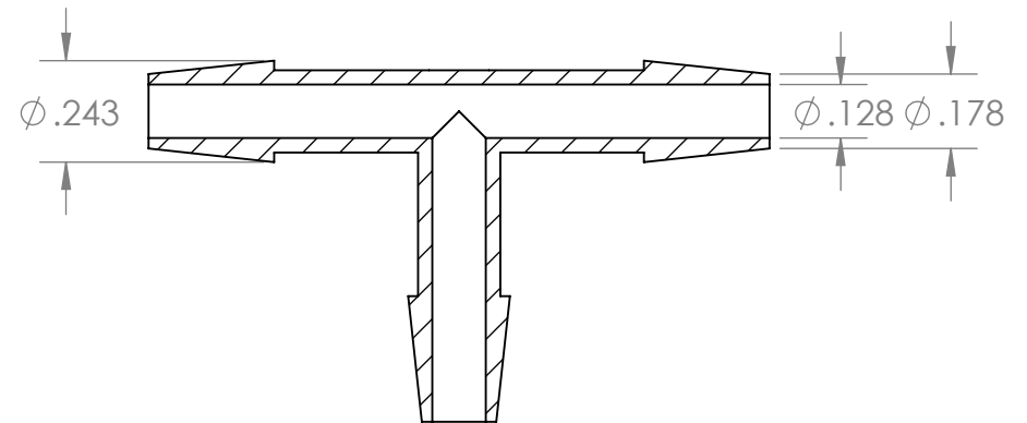
SECTION A-A
