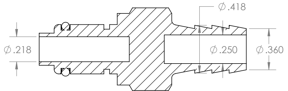
SECTION A-A SCALE 2 : 1
