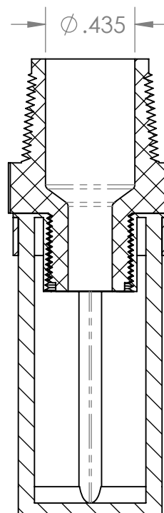
SECTION A-A SCALE 1.5 : 1
