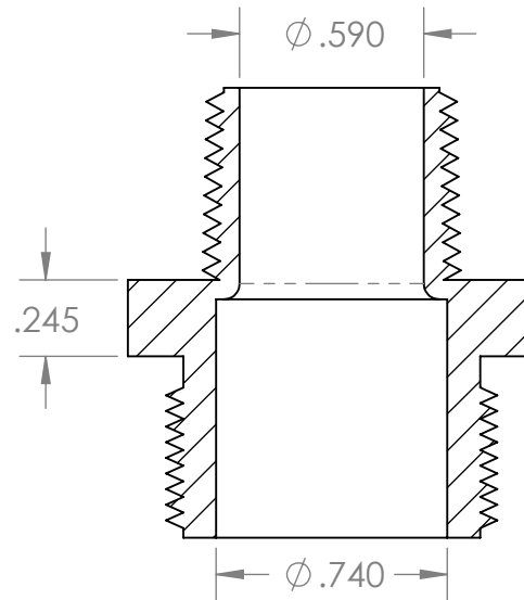
SECTION A-A SCALE 1.5 : 1
