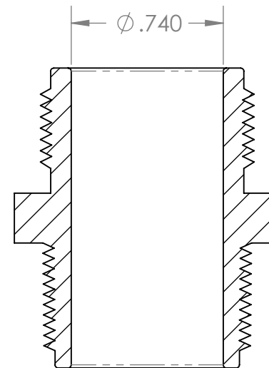
SECTION A-A SCALE 1.5 : 1
