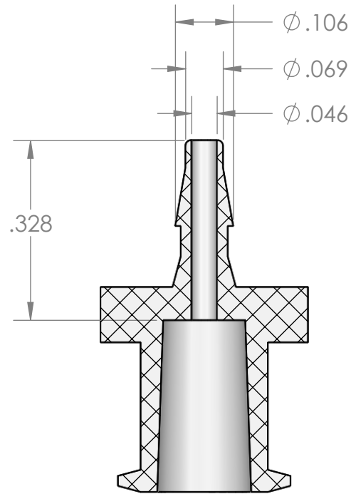
SECTION A-A
