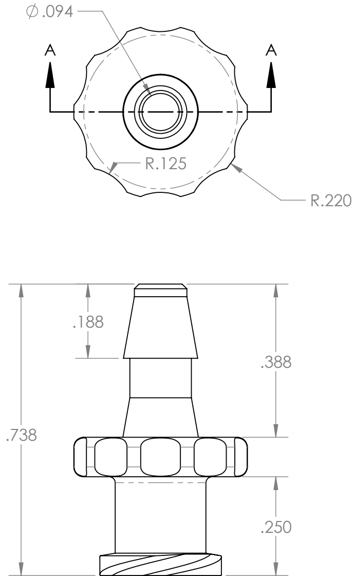
SECTION A-A
