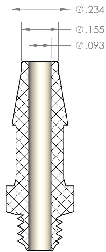
SECTION A-A
