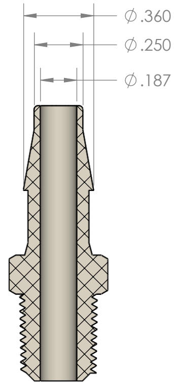
SECTION A-A
