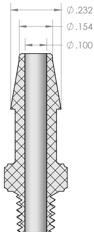
SECTION A-A
