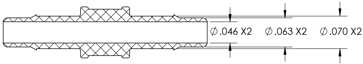
SECTION A-A
