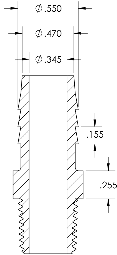
SECTION A-A
