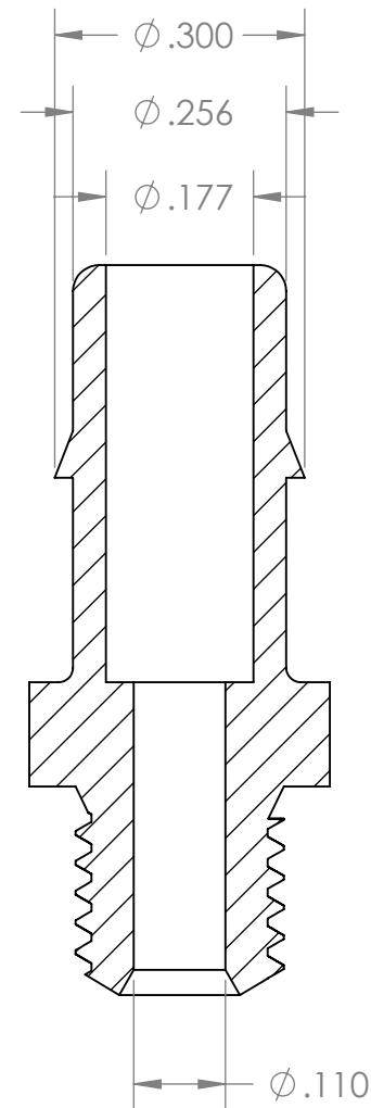
SECTION A-A
