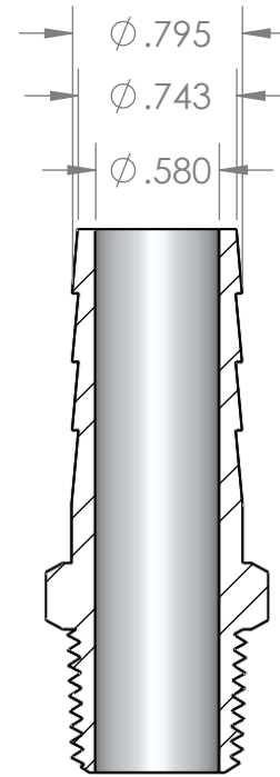
SECTION A-A
