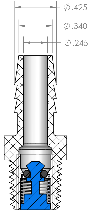
SECTION A-A
