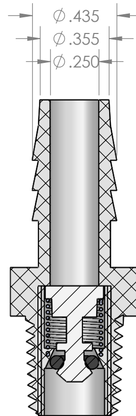
SECTION A-A
