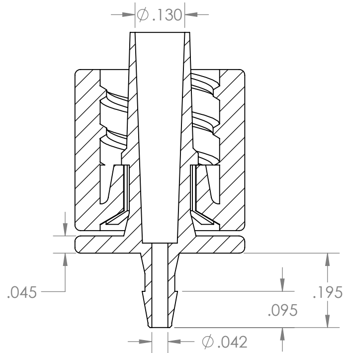
SECTION A-A
