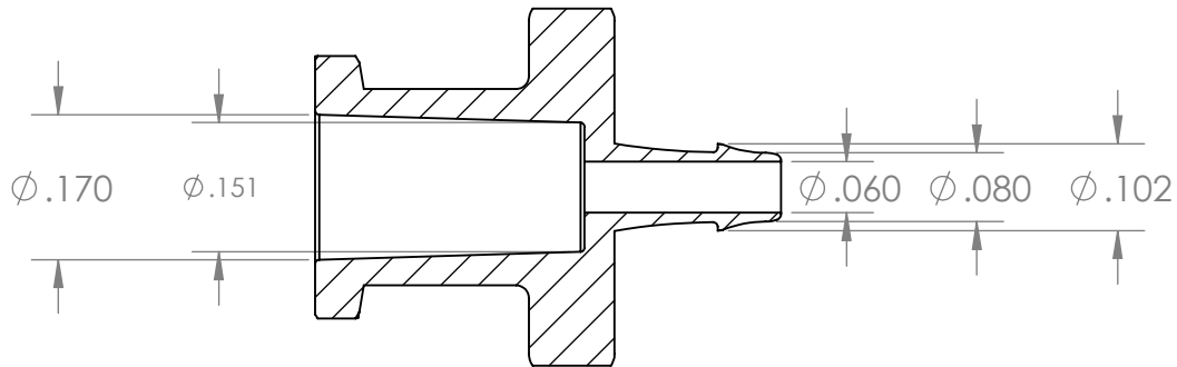
SECTION A-A
