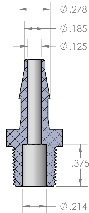
SECTION A-A
